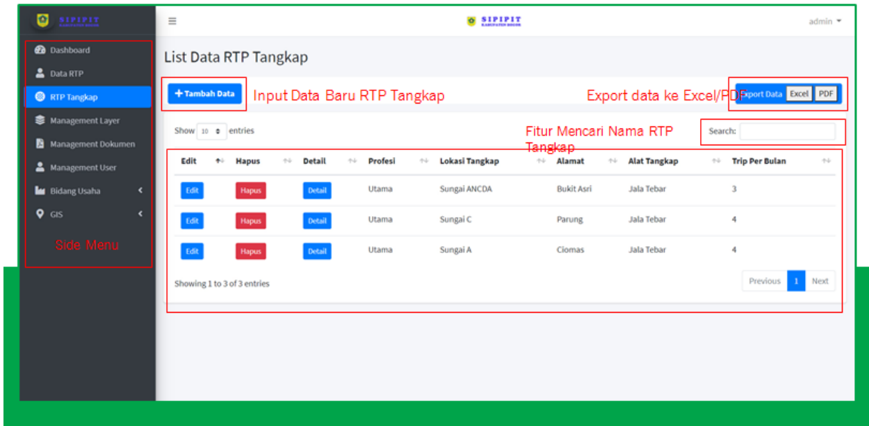
Gambar 6 Halaman List Data RTP Tangkap
